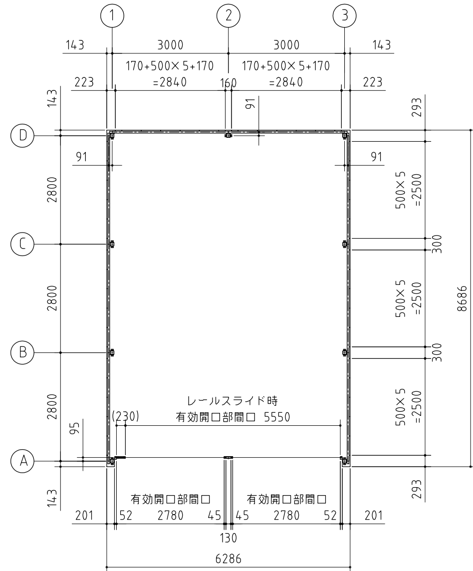
平面図
